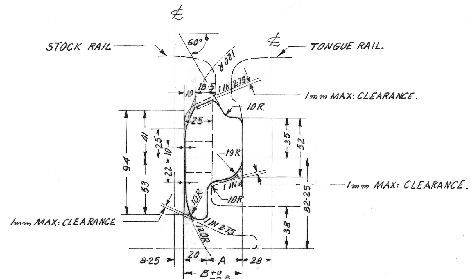
END ELEVATION X. X.
